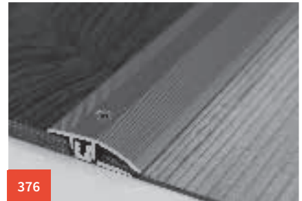
Anpassprofil Typ 376 (4-9.5mm) Breite 33mm
