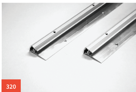
Treppenkantenprofil Typ 320 (7-16mm) Breite 23mm
